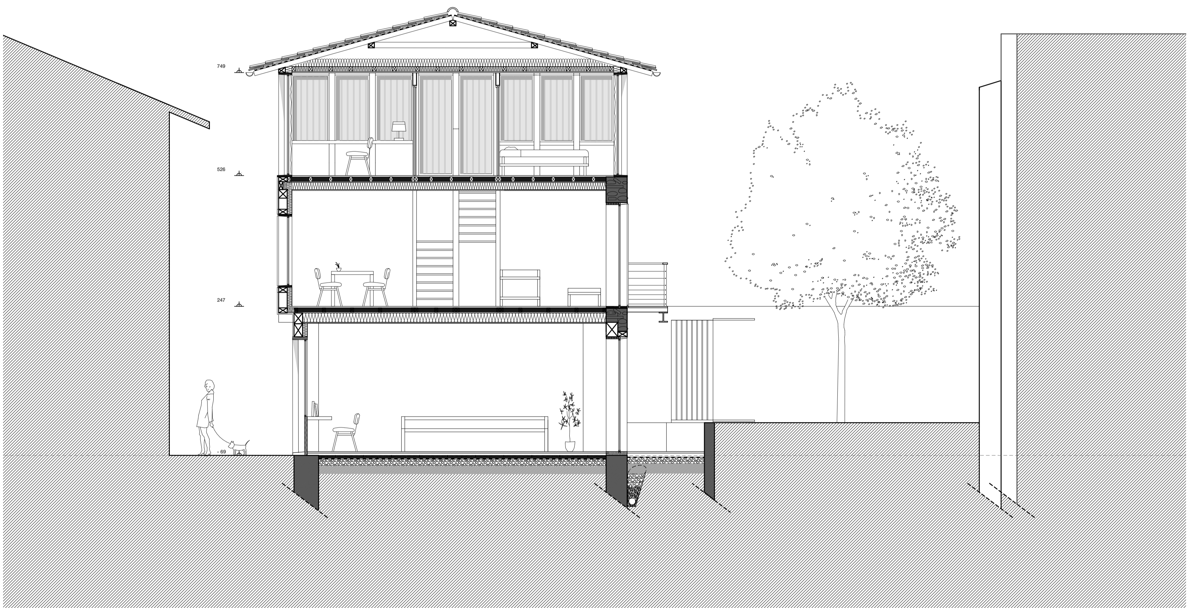
COUPE DD 1:50
