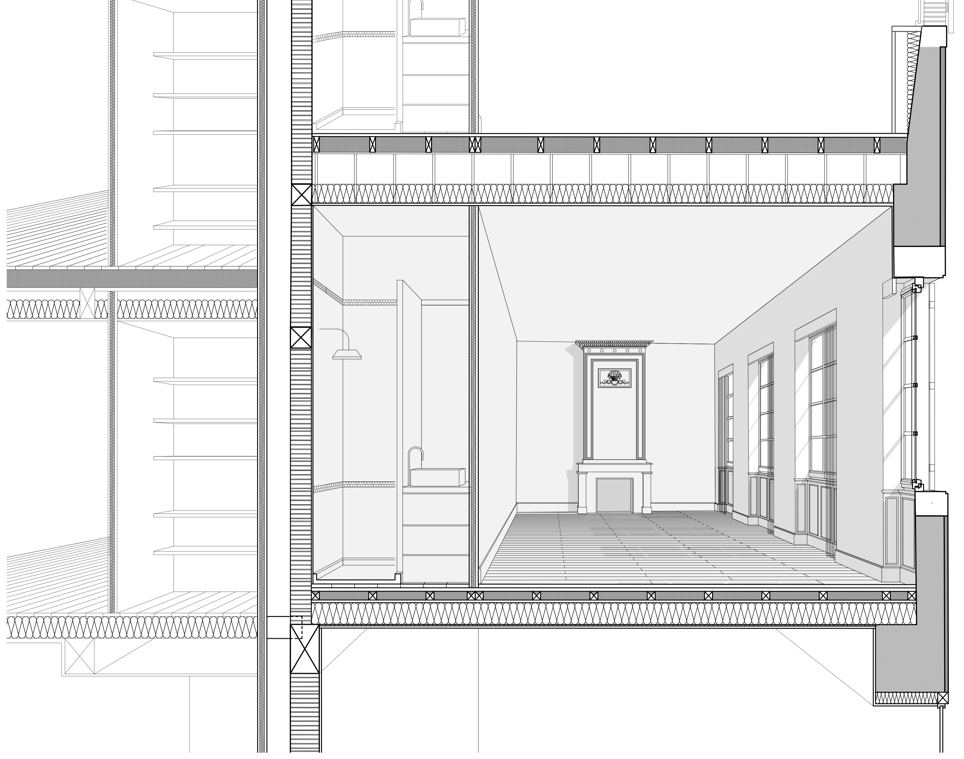
COUPE PERSPECTIVE VERS RUE JEAN JAURÈS 1:20
