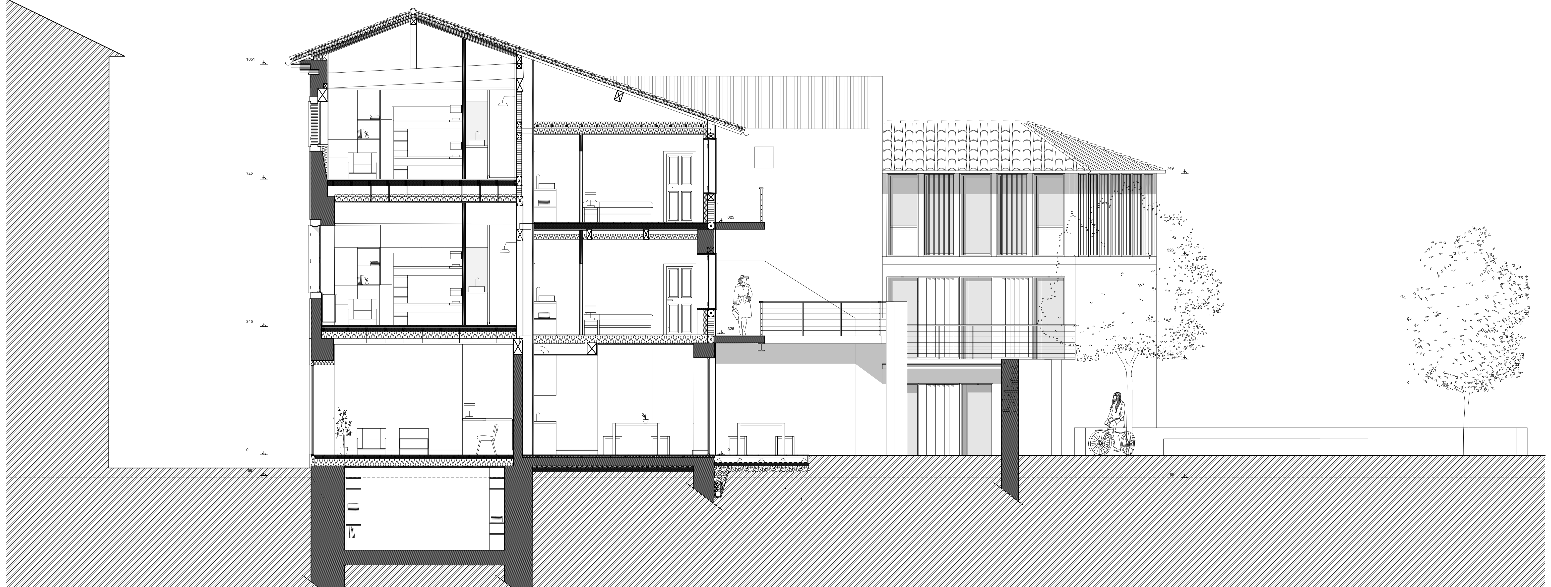
COUPE CC 1:50
