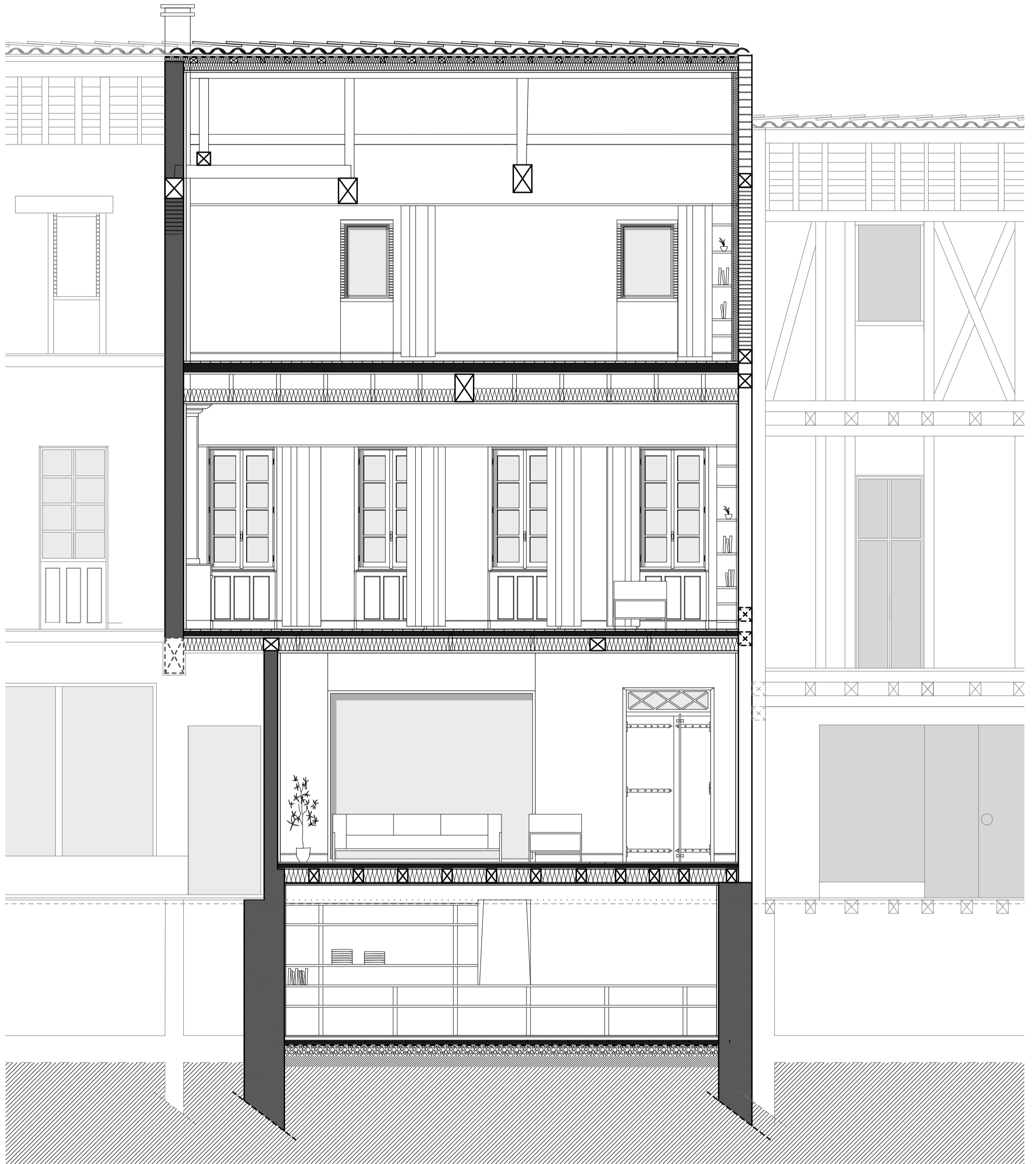
COUPE AA 1:50
